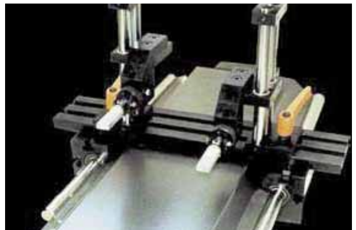
Blechbearbeitungs-Maschine mit iglidur® J Sheet metal forming machine – using iglidur® J
